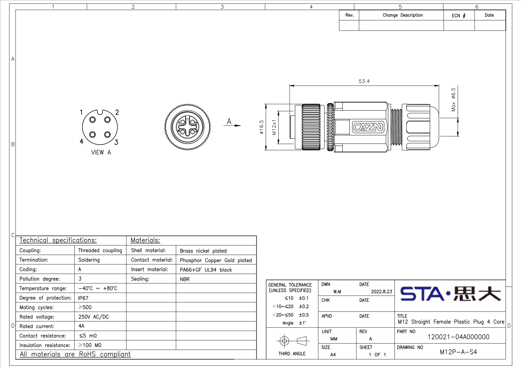
Разъём M12P-A-S4-Y — чертёж производителя
