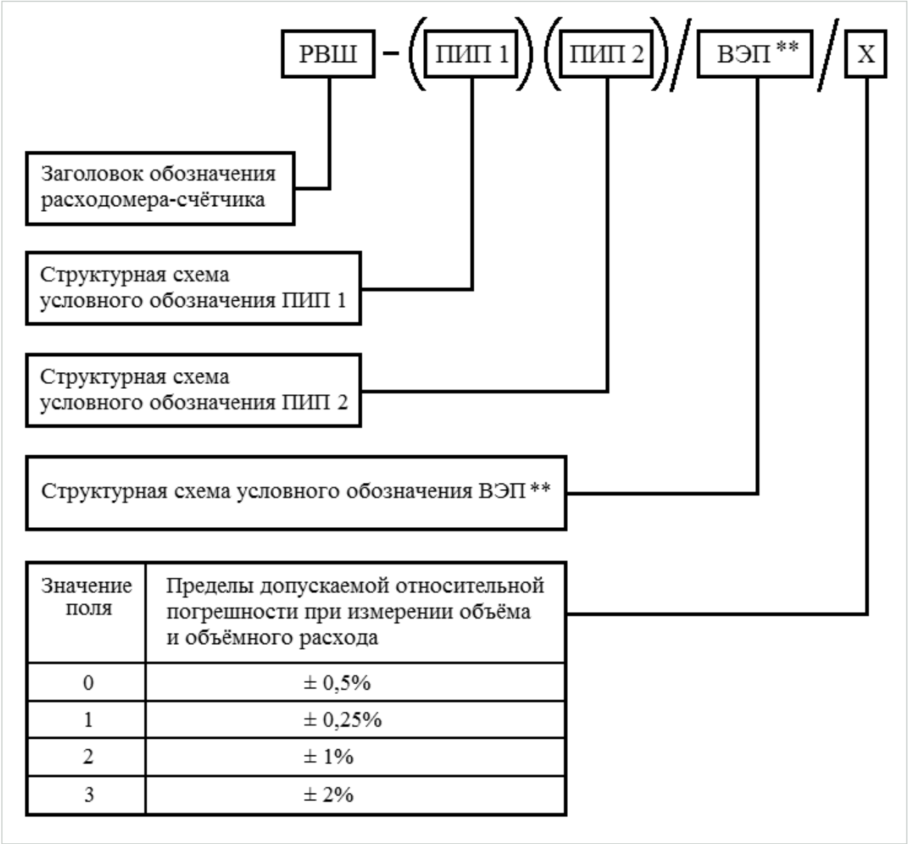
Блок-схема обозначения RVШ - двухпоточное исполнение
