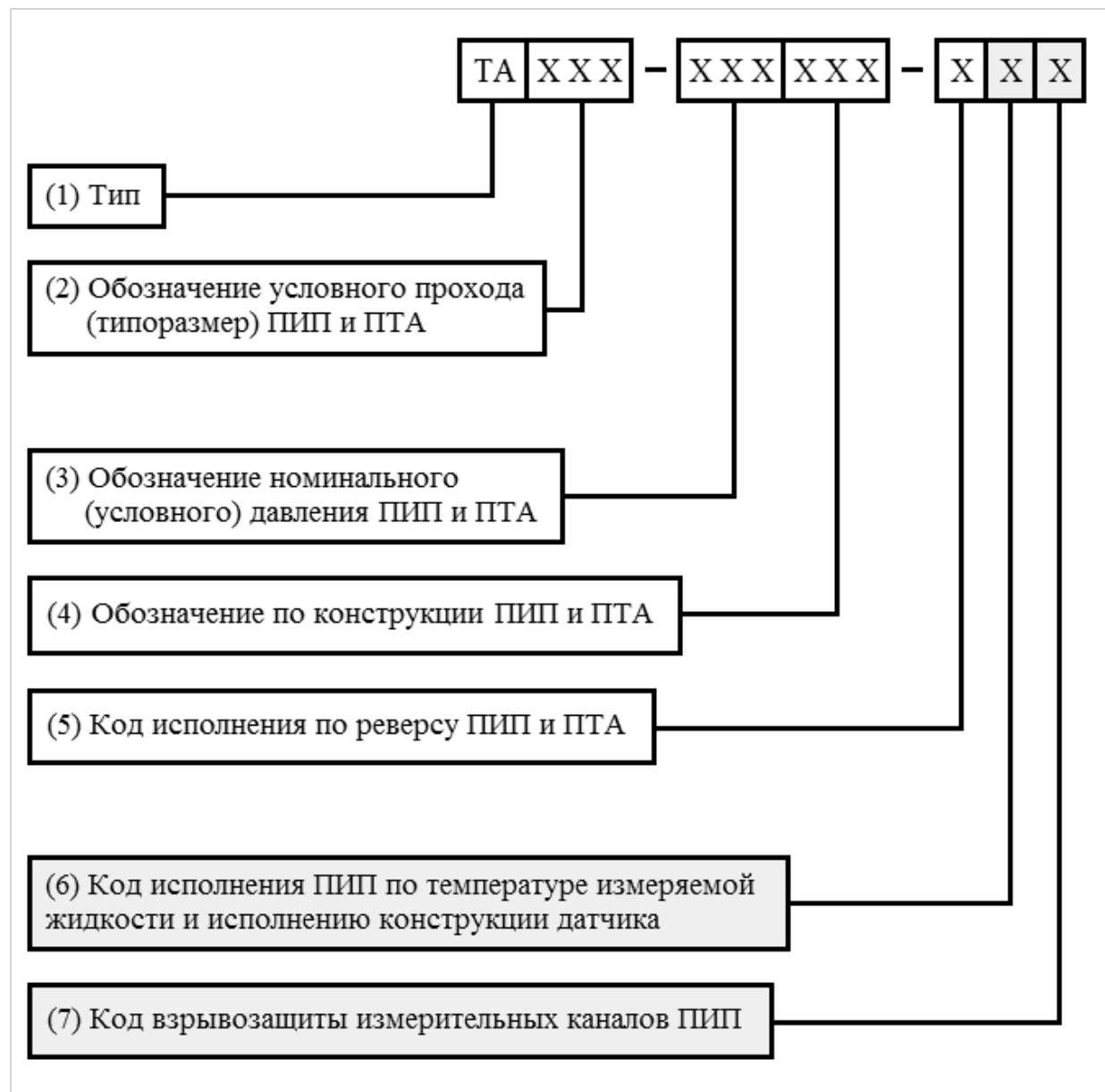
Структурная схема условного обозначения ПИП
