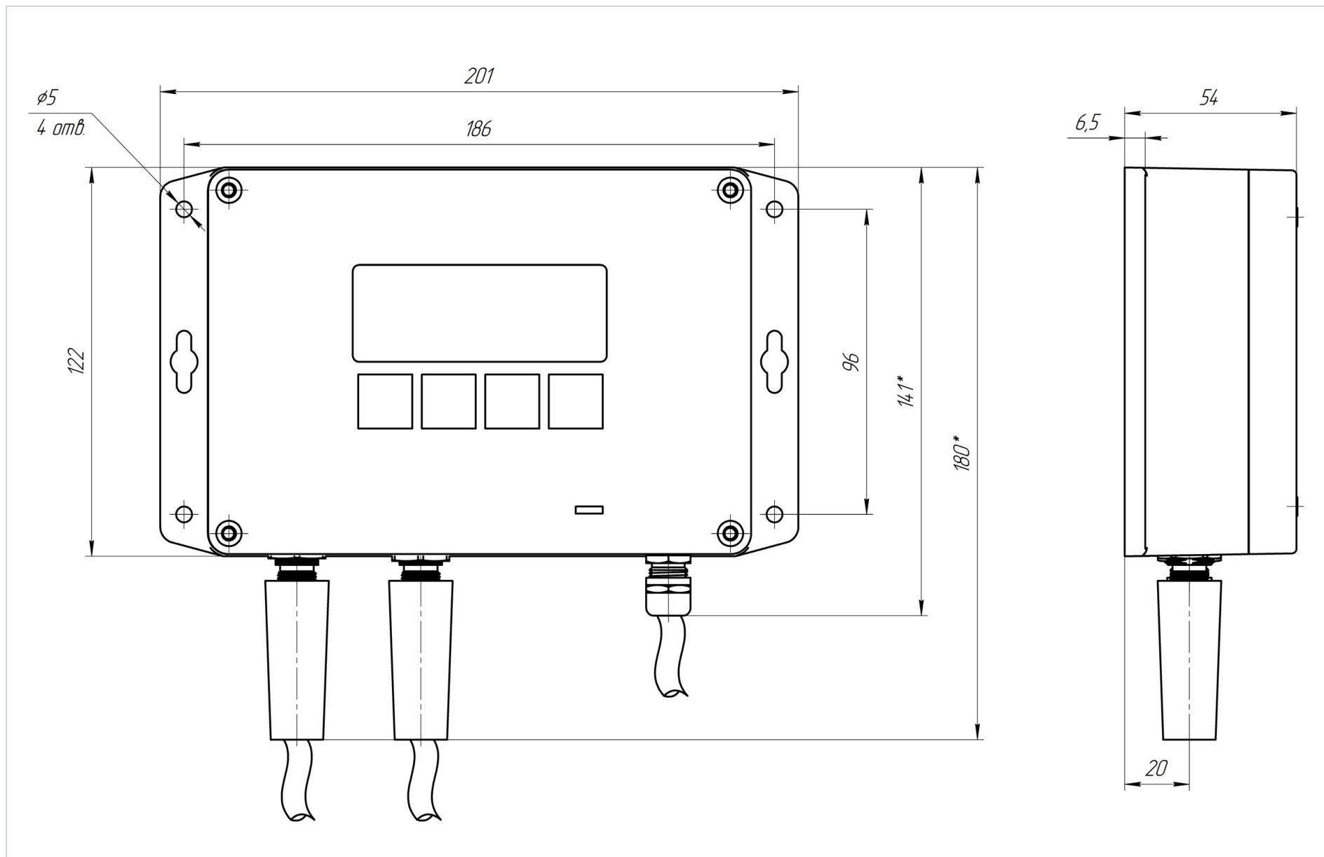
Корпус СКЭ2 — габаритно-монтажный чертёж
