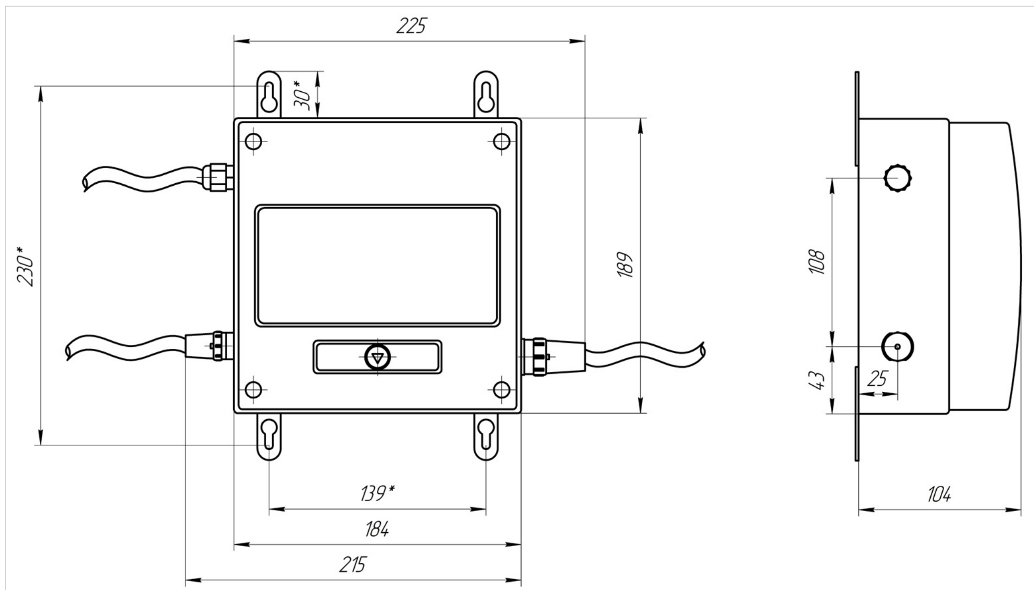
Корпус СКЭ1 — габаритно-монтажный чертёж
