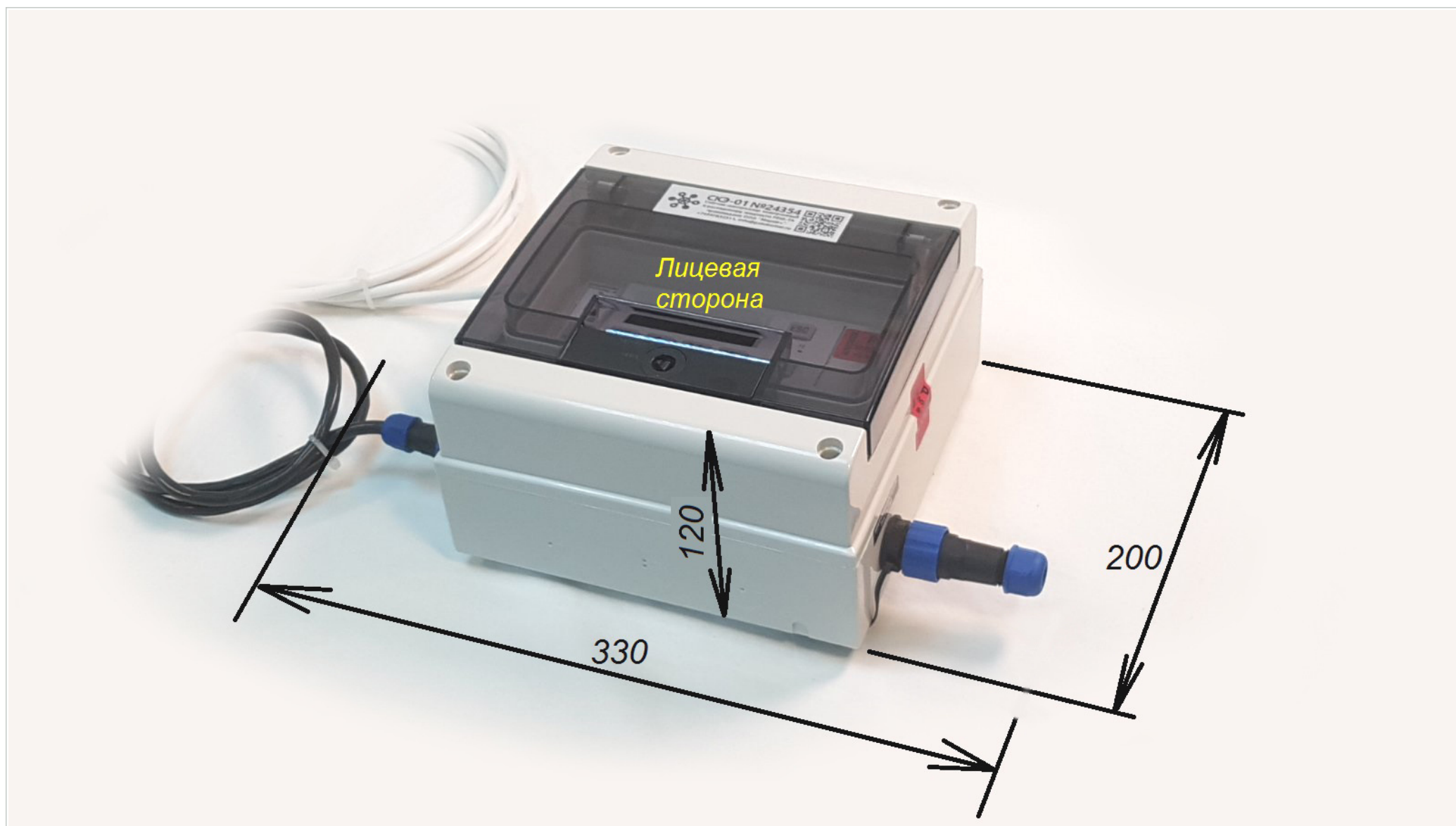
СКЭ-01 — внешние габариты
