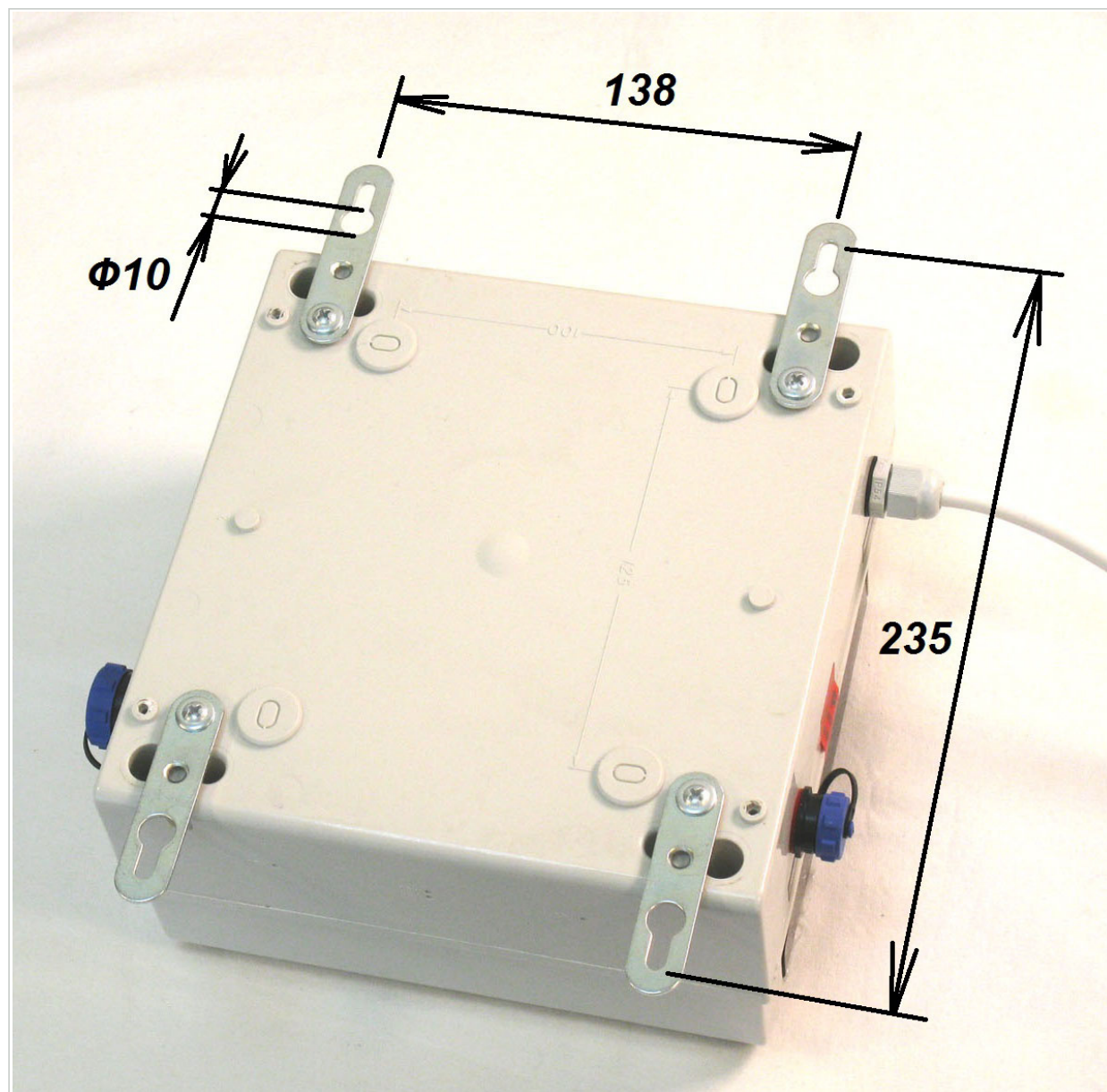
СКЭ-01 — размеры по крепёжным отверстиям
