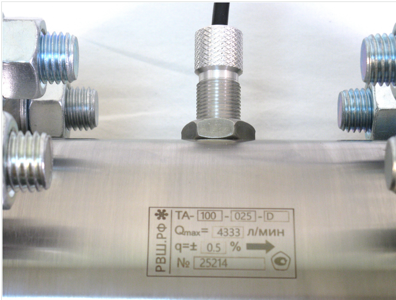
ПИП РВШ-ТА-100-D - табличка и датчик
