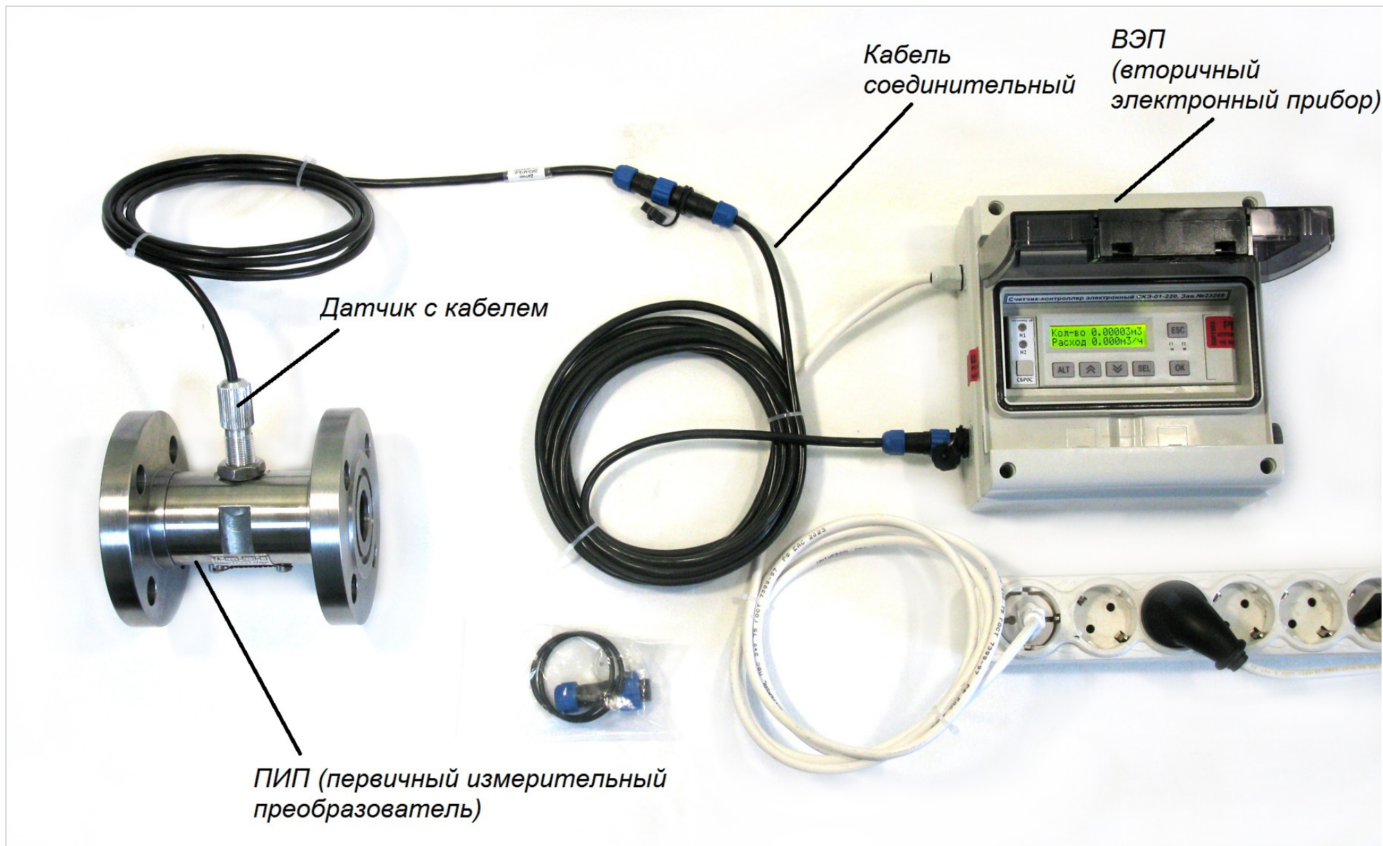
Расходомер-счётчик РВШ-ТА
