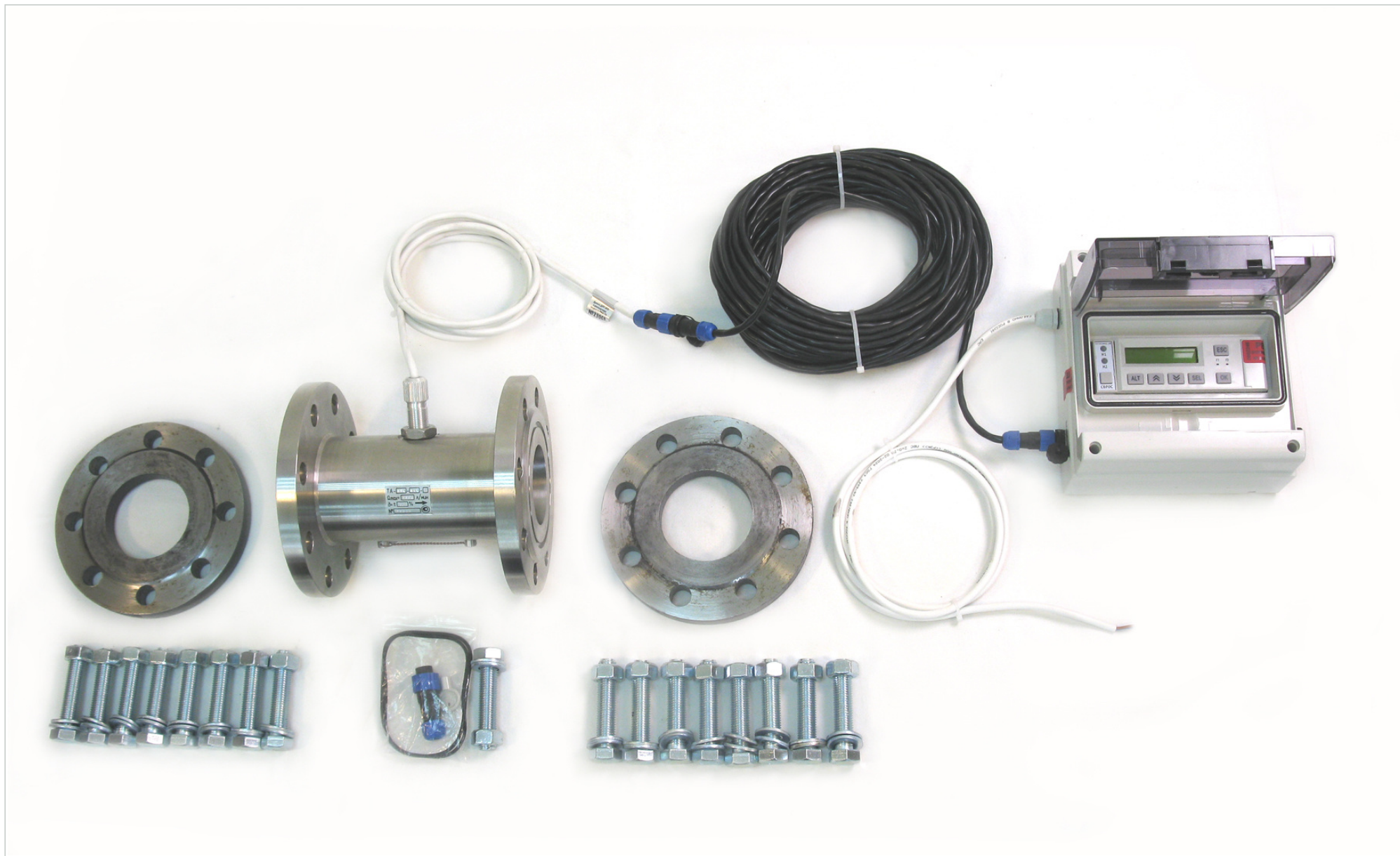
ТА-065-025-D с ДИЭ-М18-И, СКЭ-01-024 и КМЧ
