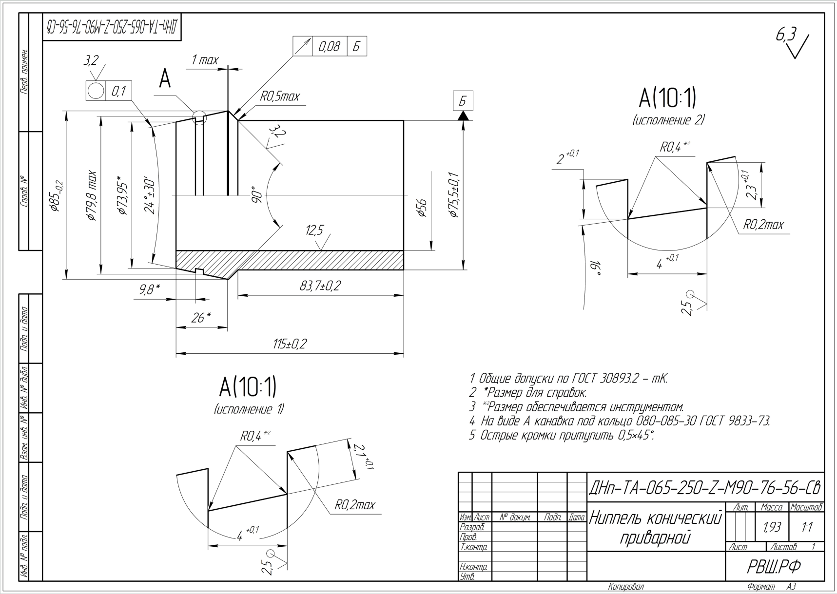
Ниппель ДНп-ТА-065-250-Z-M90-76-56-Св
