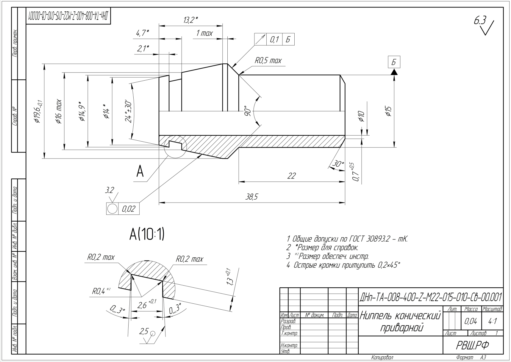
Ниппель ДНп-ТА-008-400-Z-M22-015-010-Св-00.001
